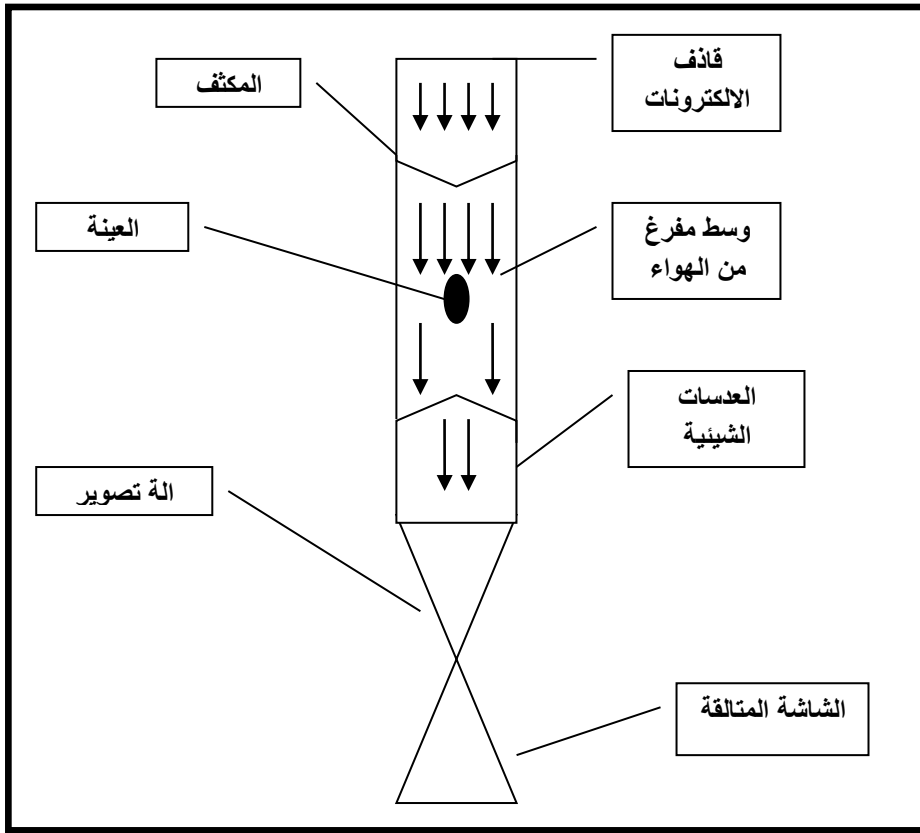
اساس عمل المجهر الالكتروني
